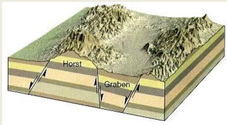
priekopová prepadlina hrásť
