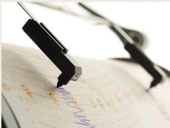
zemetrasenie na Haiti
