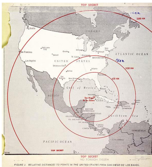
Obr. 2 - dostrel sovietskych rakiet z Kuby (zdroj: www.nationalarchives.gov.uk )
